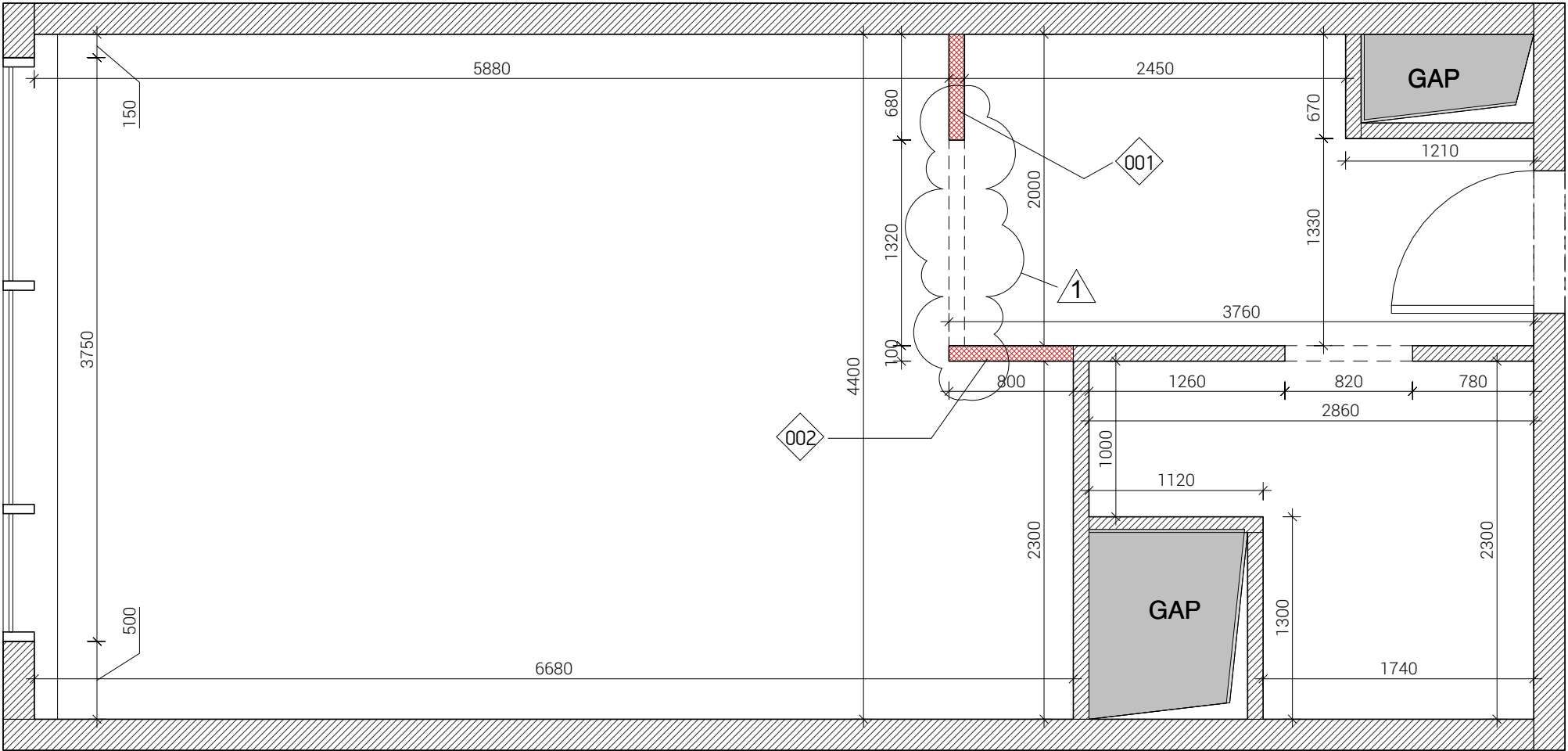
A | გეგმა / დგომნათქო მ1 : 50
