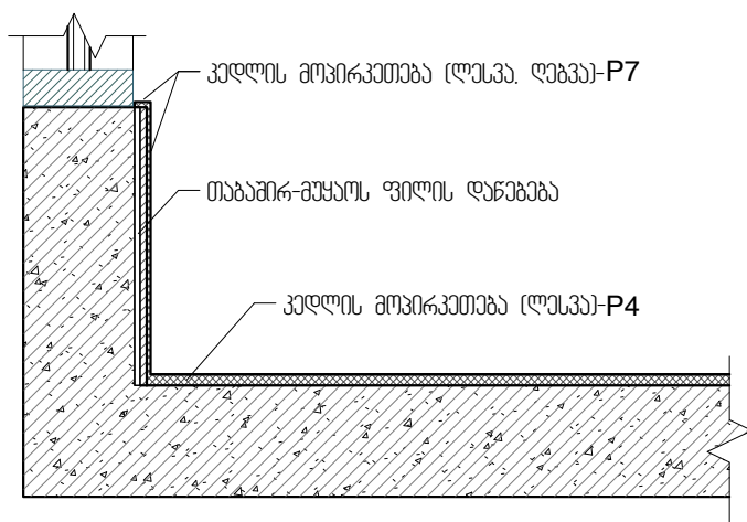
A | ფრაგმენტი 3 მ 1 : 20
