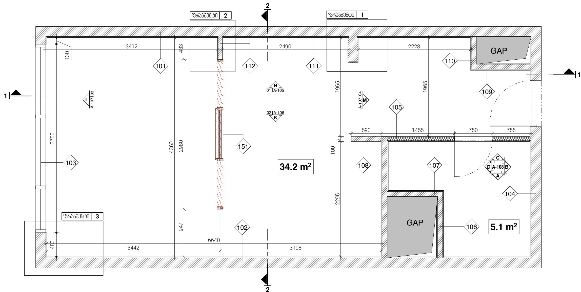
A | გეგმა მ 1 : 50
