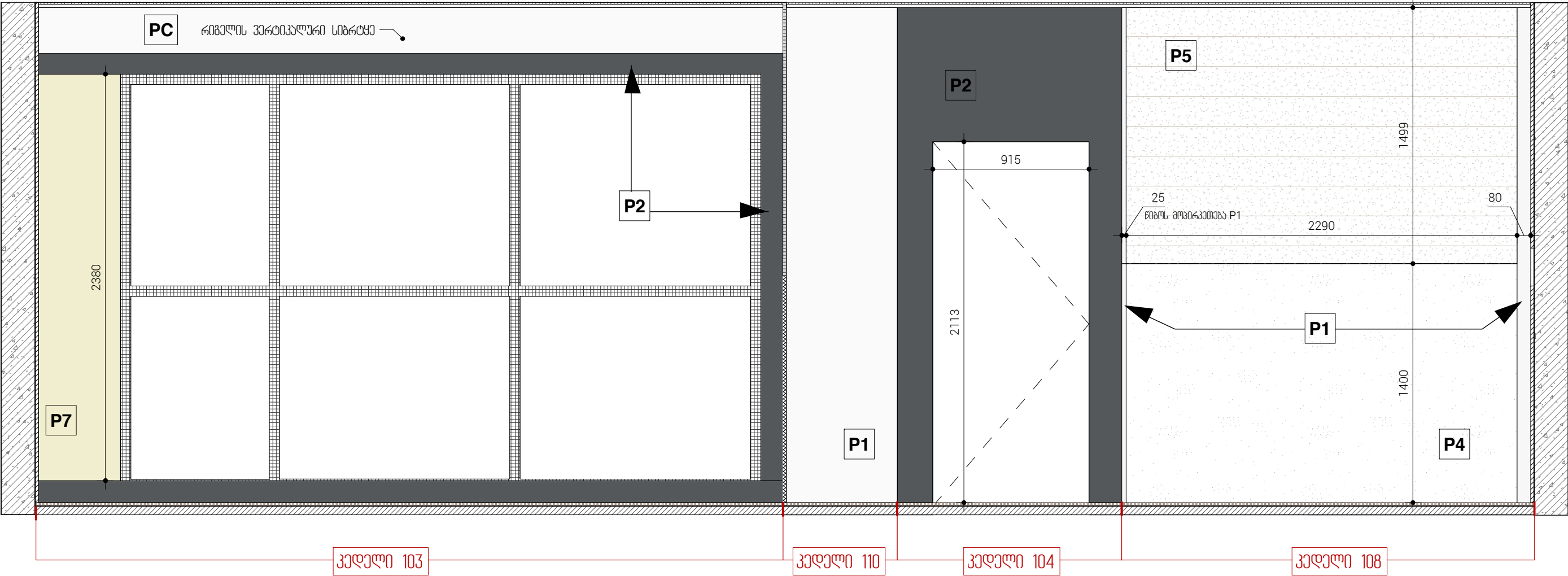
03 | განშლ- L მ 1 : 25
