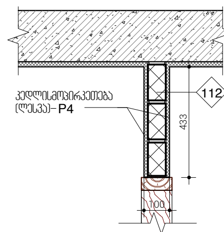
A | ფრაგმენტი 2 მ 1 : 20
