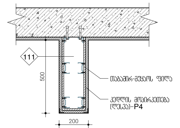
A | ფრაგმენტი 1 მ 1 : 20
