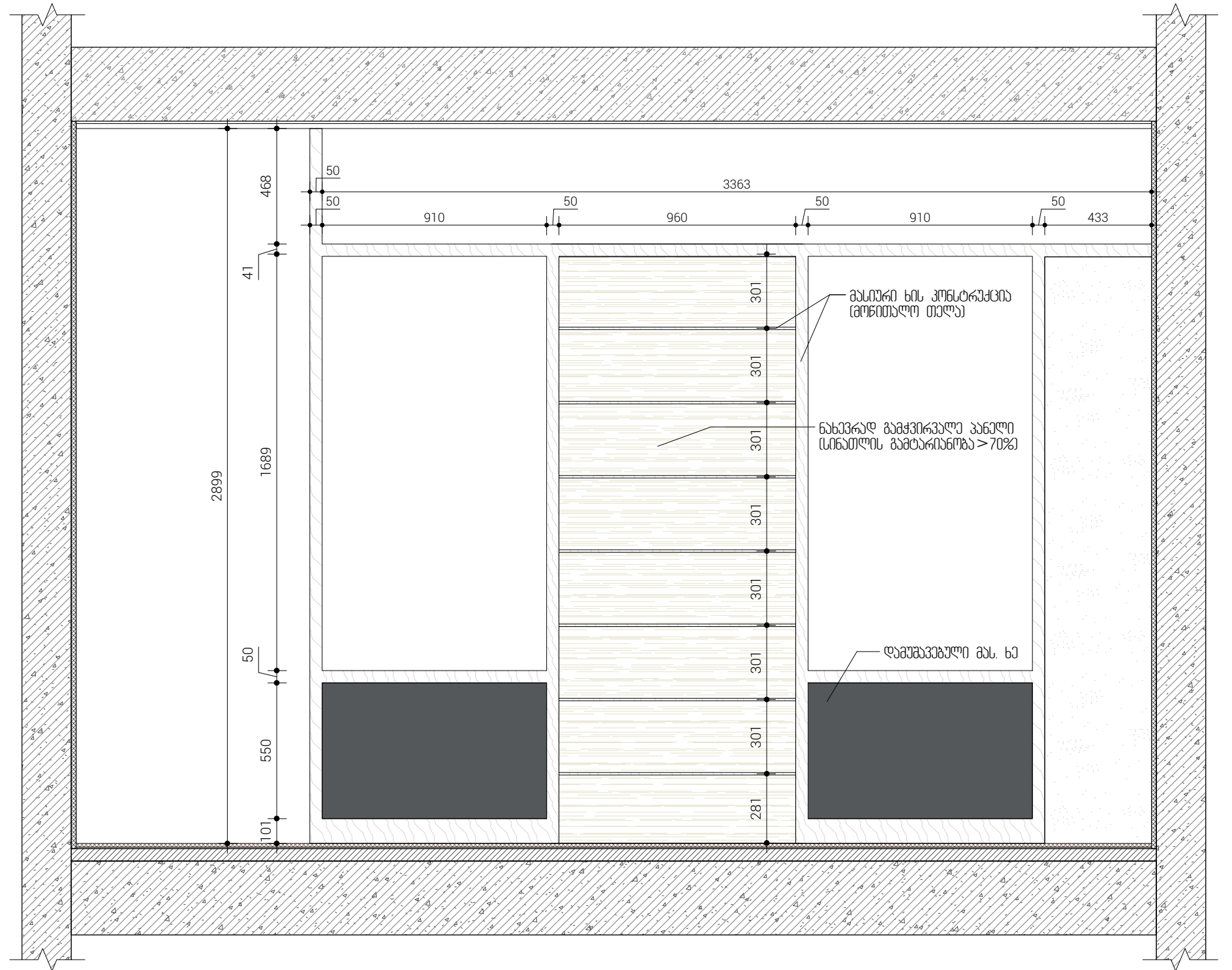
S | ჭრილი 2-2 მ 1 : 20
