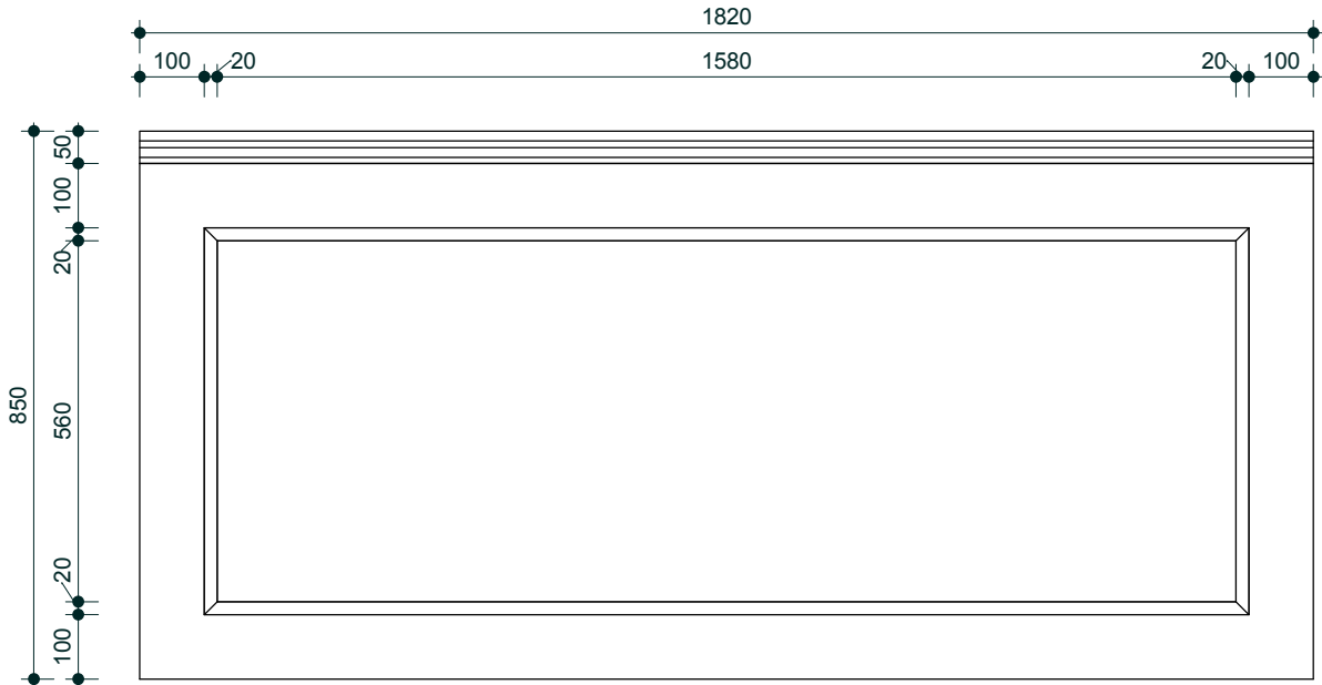
პანელის ფასადი მ 1/10
