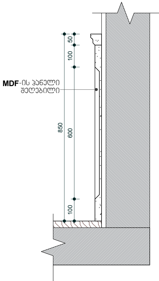
ღებელი: C-C მ 1/10
