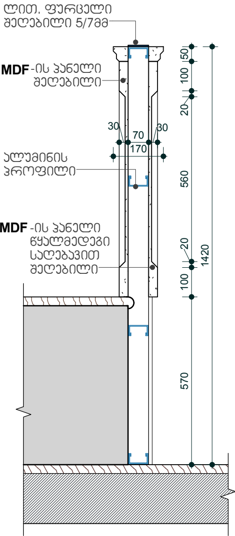
ღირსეულობა: A-A მ 1/10
