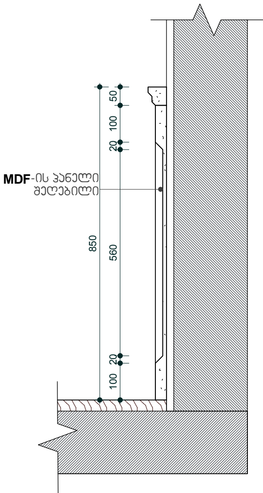
ღებელი: D-D მ 1/10
