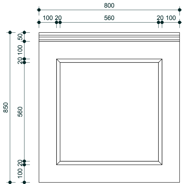
პანელის ფასადი მ 1/10
