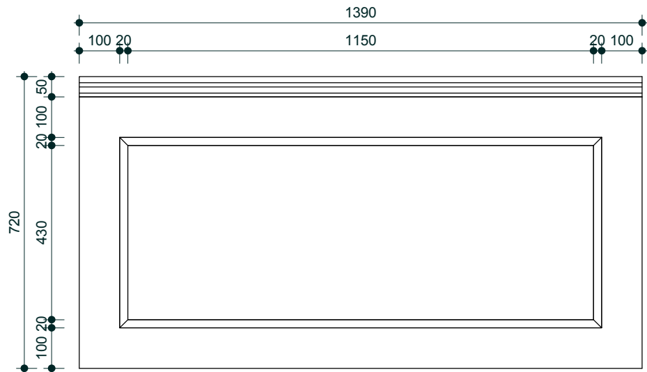
პანელის ფასადი მ 1/10
