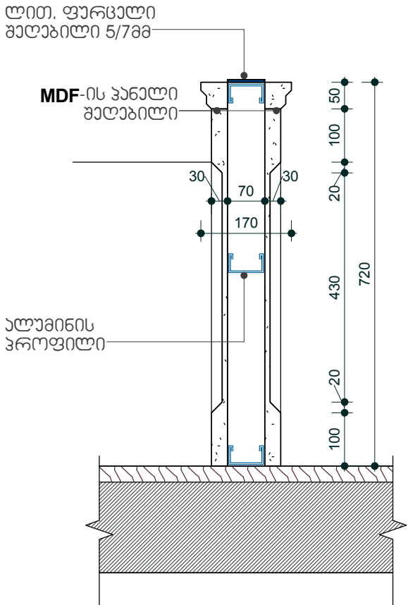
ღებულობა: B-B მ 1/10
