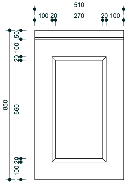
პანელის ფასადი მ 1/10
